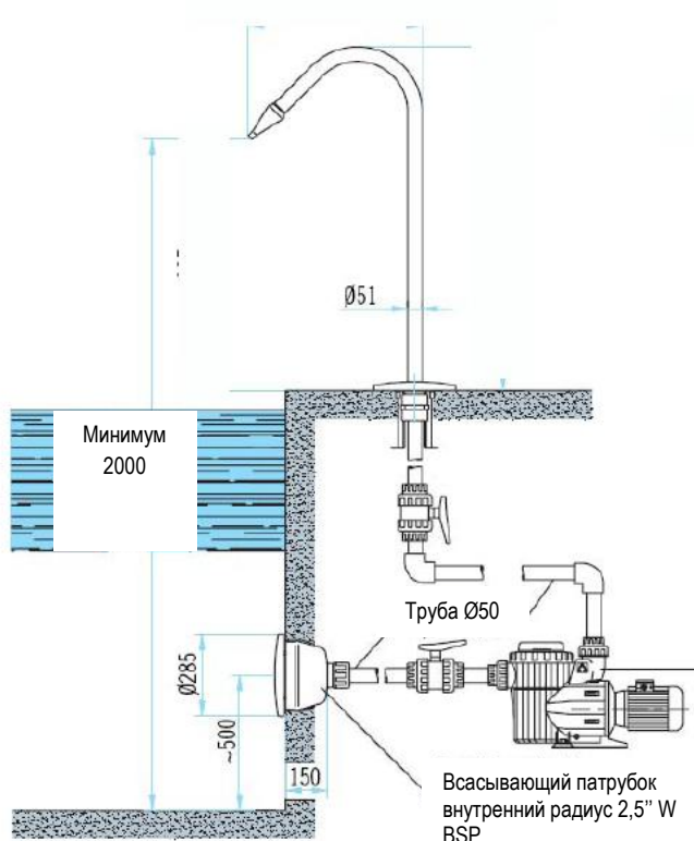
форсунка 1 код 05572
